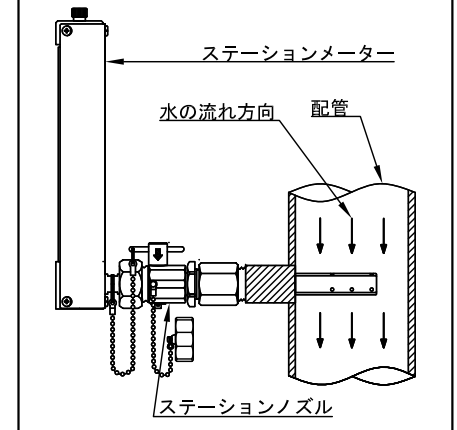
ステーションメーター取付概略図
