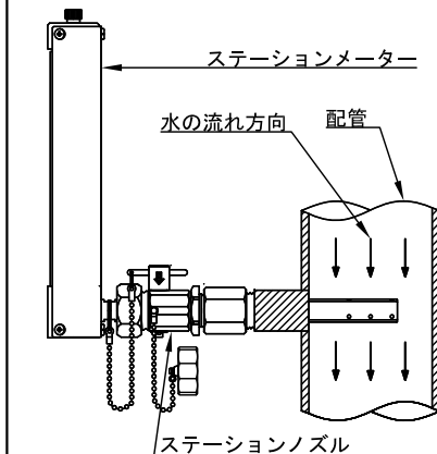
ステーションメーター取付概略図
