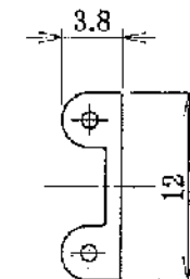
断面A-A(2:1)
