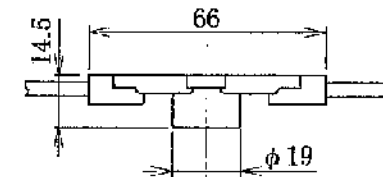
B矢視図(1:2)
