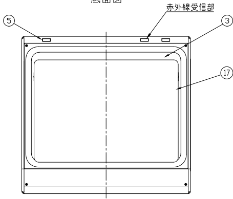
底面図
