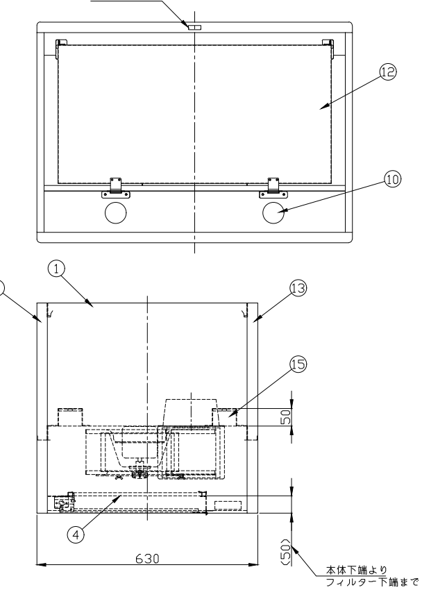
底面図
