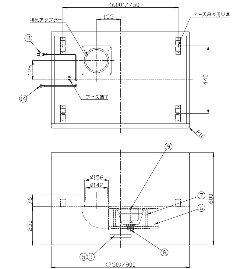
底面図
