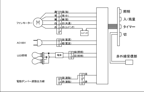
□結線図
