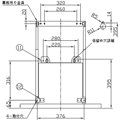
背面取付図
