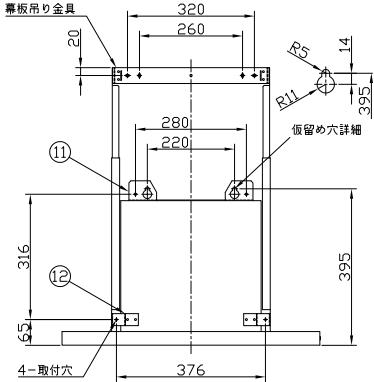
背面取付図
