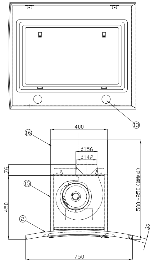
底面図
