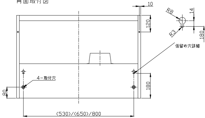
背面取付図
