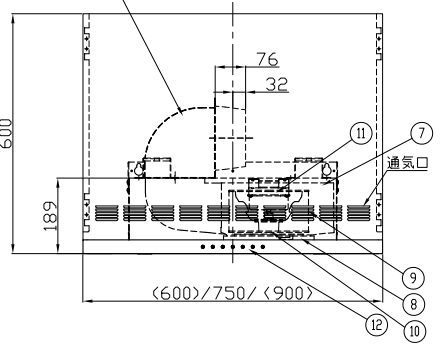
側方排気の場合 (別売エルボ使用)
