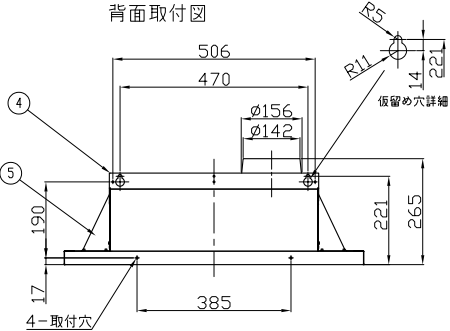
背面取付図
