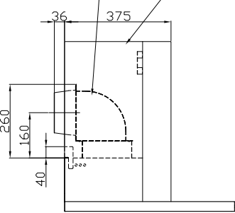
後方排気の場合 (別売アップエルボ使用)
