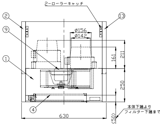
名称 デザインフード外観図
