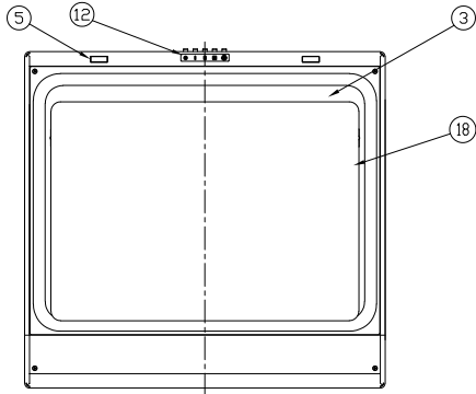
底面図
