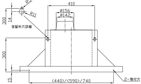
背面取付図
