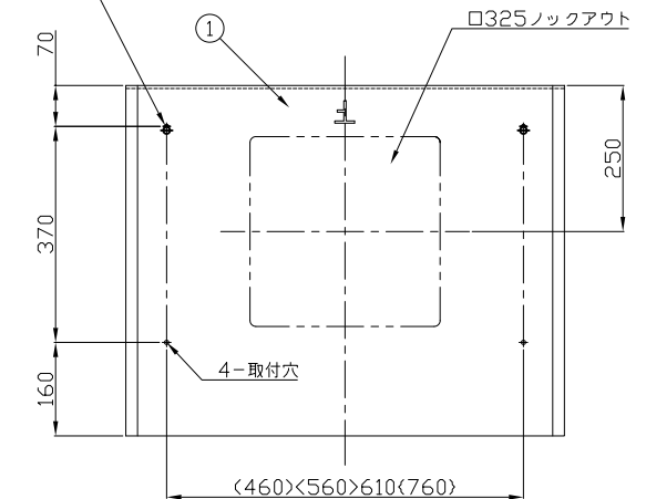
背面取付図
