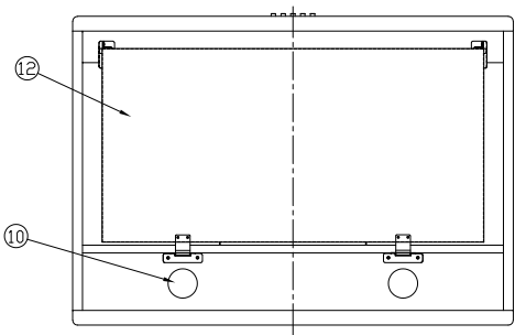
底面図
